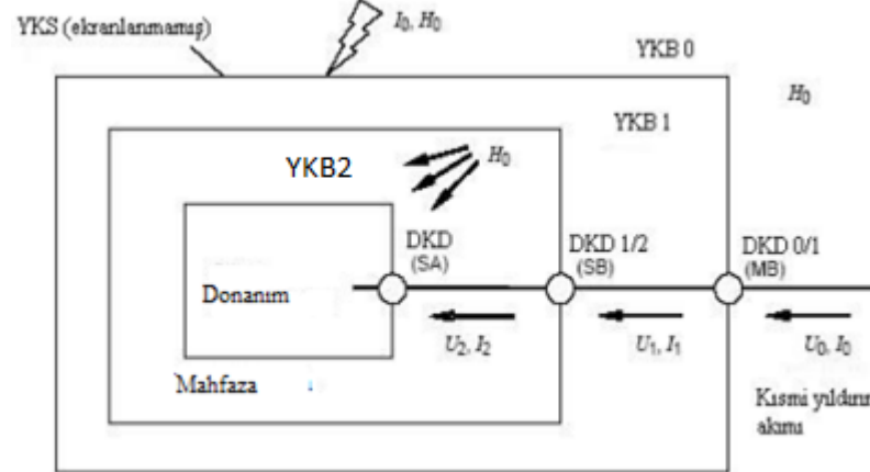
Şekil 7.5c- – YKB 1 girişinde DKD koruması yapılan ve iç hatları ekranlanan YEKS – Donanım, iletilen darbelere karşı korunmuştur ( U_2 \ll U_0 ve I_2 \ll I_0 ) ve ışınlama yayılan manyetik alanlara karşı da korunmuştur ( H_2 \ll H_0 )
