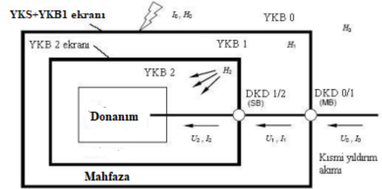
Şekil 7.5a- Hacimsel ekranlama ve koordineli DKD sistemi kullanan YEKS – Donanım, iletilen darbelere karşı korunmuştur ( U_2 \ll U_0 ve I_2 \ll I_0 ) ve ısınlımla yayılan manyetik alanlara karşı da korunmuştur ( H_2 \ll H_0 )
