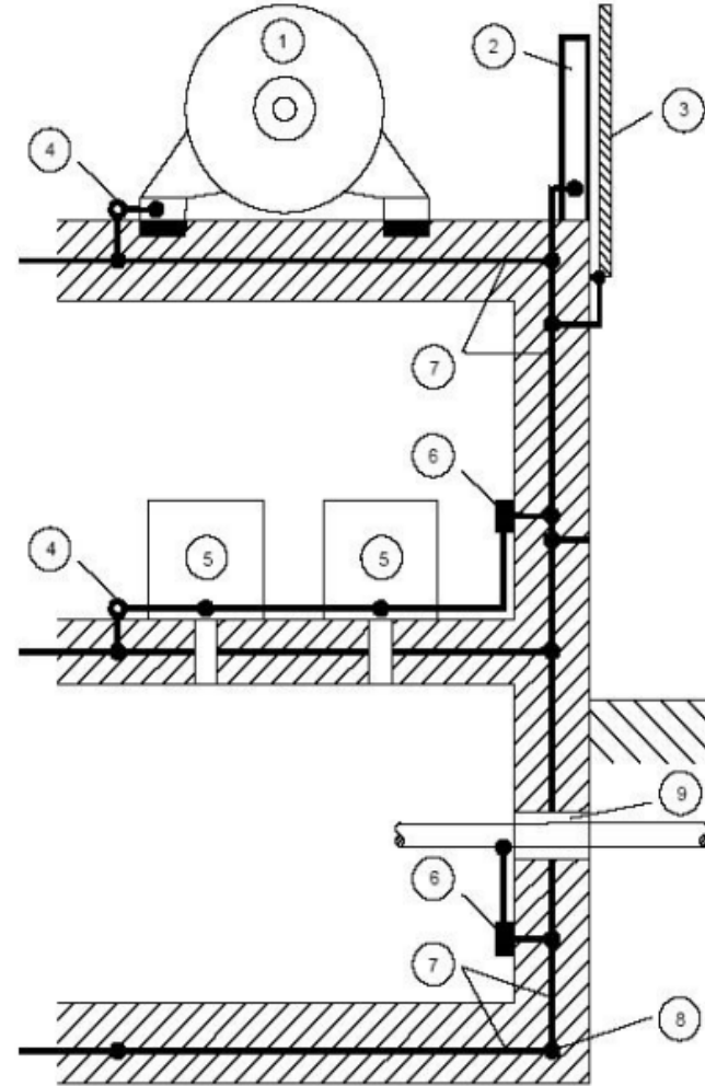
Şekil 7.10-Bir yapının donatı çubuklarının, yıldırımın elektromanyetik darbesine karşı koruma önlemi ve eş potansiyel kuşaklama amacıyla kullanılması
