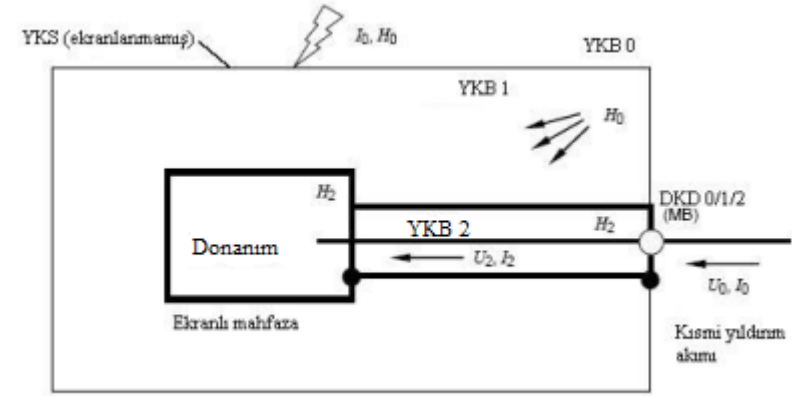
Şekil 7.5c- – YKB 1 girişinde DKD koruması yapılan ve iç hatları ekranlanan YEKS – Donanım, iletilen darbelere karşı korunmuştur ( U_2 \ll U_0 ve I_2 \ll I_0 ) ve ışınlama yayılan manyetik alanlara karşı da korunmuştur ( H_2 \ll H_0 )
